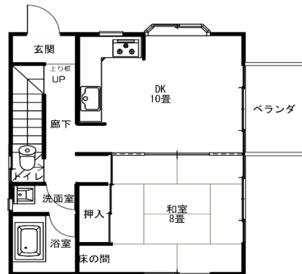
1階 縮尺 1/100
