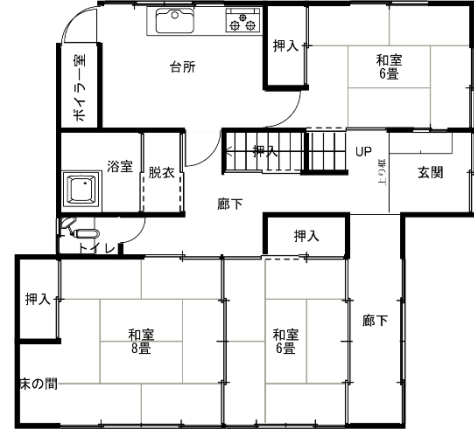
1 階 縮尺 1/100
