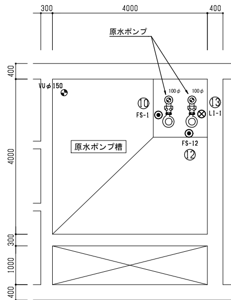
原水ポンプ槽平面図 S=1/50
