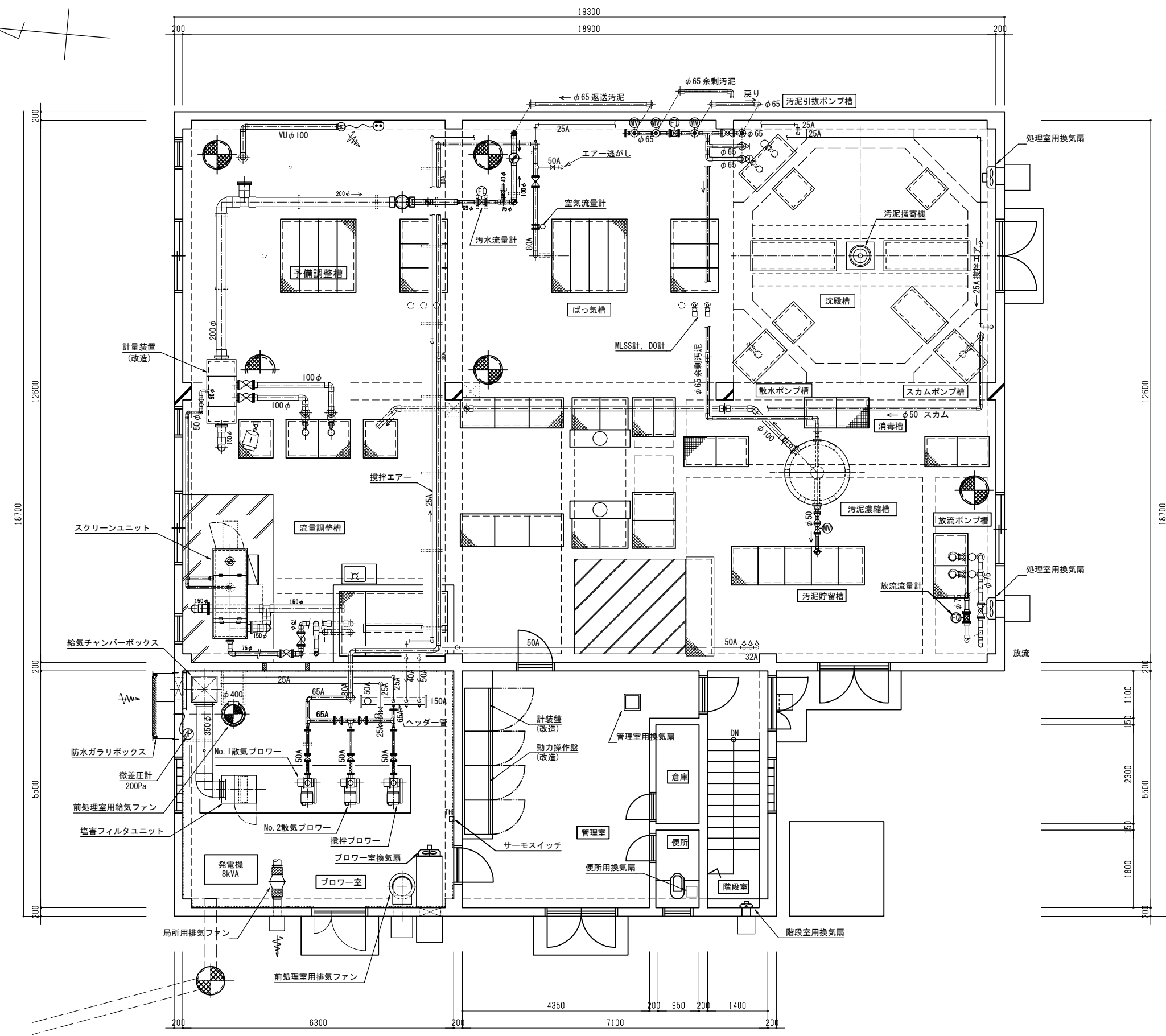
上部平面図 S=1/50
