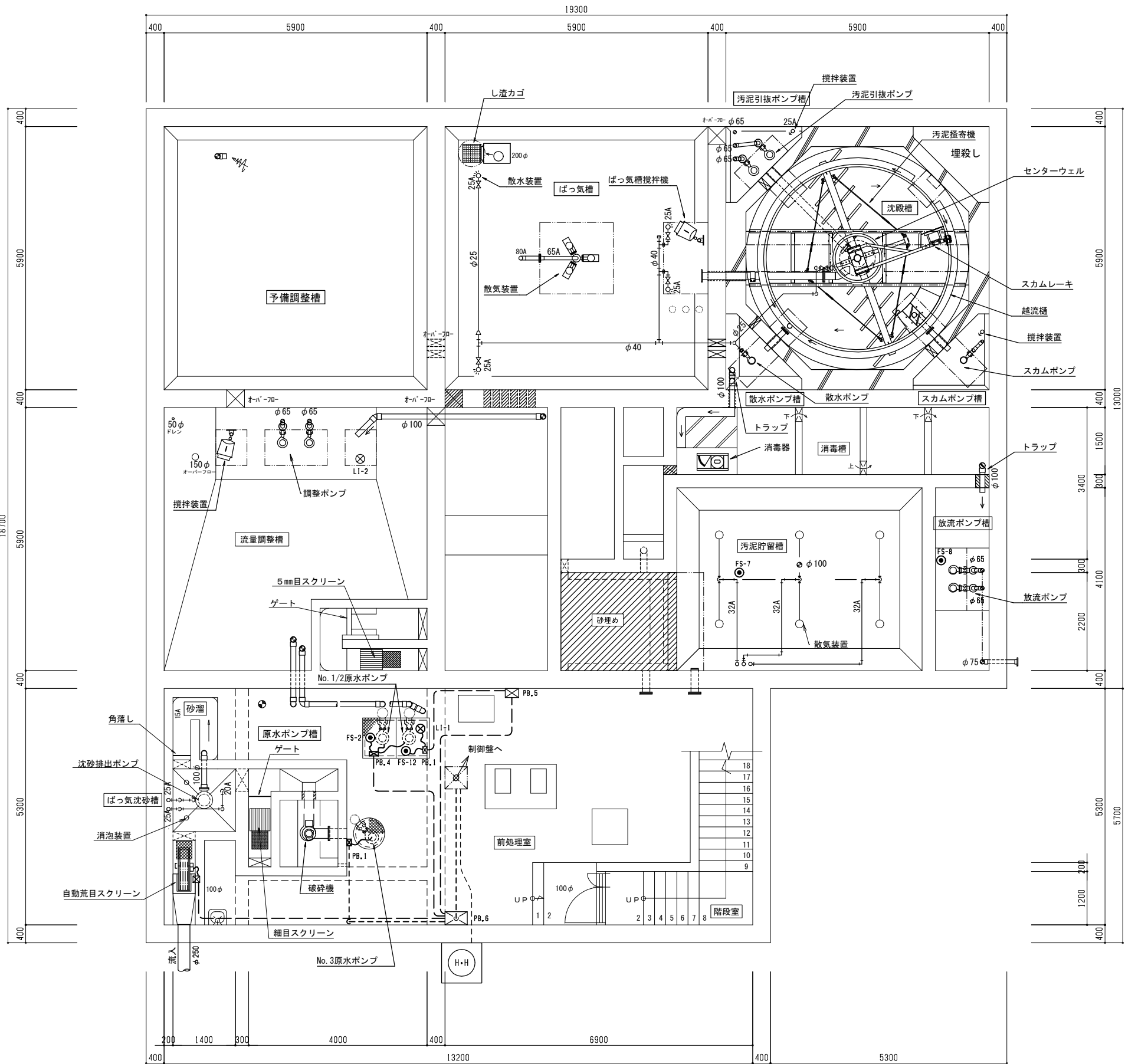
下部平面図 S=1/50
